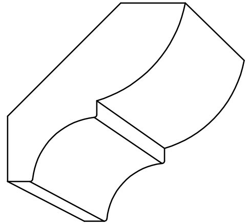
CR 2562 - 11/16" x 2-9/16" P=1-13/16" - D=1-13/16"
