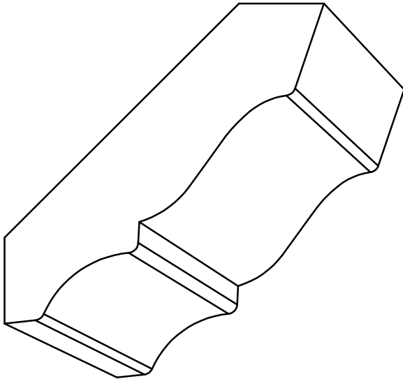
CR 3375 - 3/4" x 3-3/8" P=2-3/8" - D= 2-3/8"
