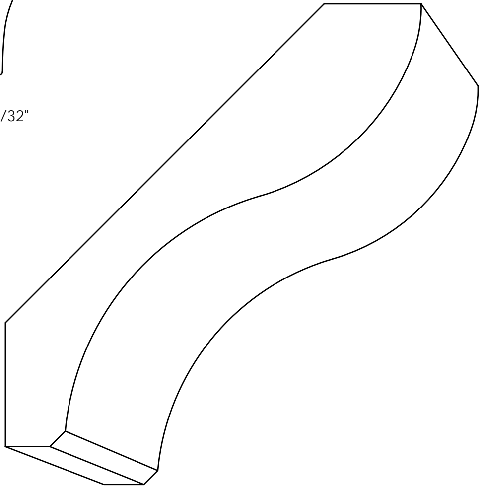
CR 6375 - 1-1/4" x 6-3/8" P=4-3/8" - D=4-5/8"
